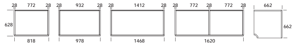
3- ANTA SCORREVOLE 3 SETTORI. SLIDING DOOR WITH 3 SECTIONS. PUERTA CORREDERA 3 SECTORES.
