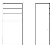
settimanale L 66 P 48 H 130 6-drawer tallboy sinfonier 6 cajones
