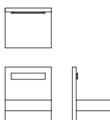
comodino sospeso L 60 P 52 H 77 wall-mounted bedside table (mesita montada en la pared)
